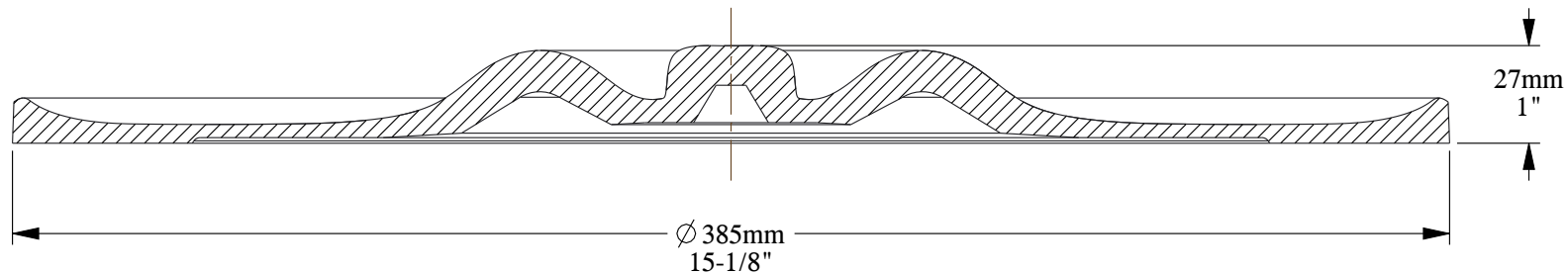
SECTION A-A SCALE 1:2
